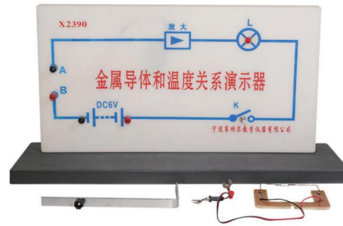
▲ X2390 金属导体和温度关系演示器
