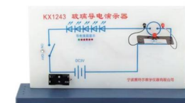
▲ KX1243 玻璃导电演示器
