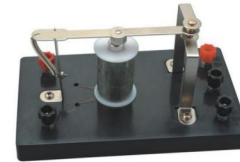
▲ 24014 外演示电磁继电器
