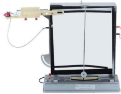
▲ J2188 二维空间-时间描述仪
