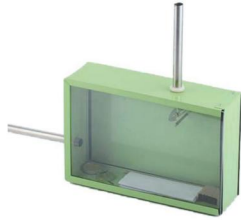
▲ J253 风的形成演示箱
